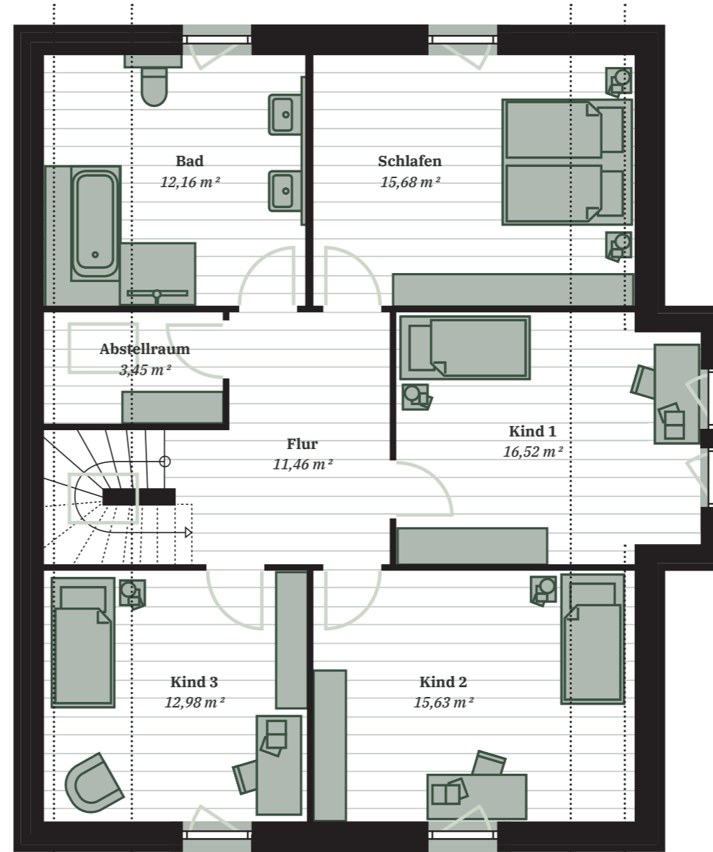
DACHGESCHOSS
